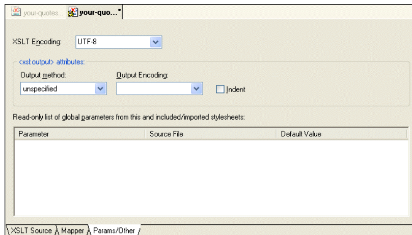
Figure 23. Specify XSLT Parameters Here or in XSLT Source
